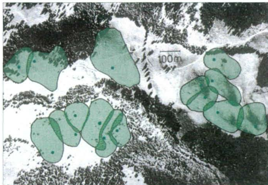
Abb. 13: Luftbild der Königsbach- und Büch- senalm im Nationalpark Berchtes- gaden (D) mit den Territorien der dort ansässigen Murmeltierfamilien (Freiga- be des Fotos durch Regierung von Oberbayern G7/88995). Die Familien- territorien sind durchschnittlich etwa 2,5 ha groß. Die Überlappungsbereiche benachbarter Territorien sind schraff- tiert gekennzeichnet, die Lage der Winterbaue mit Punkten.
