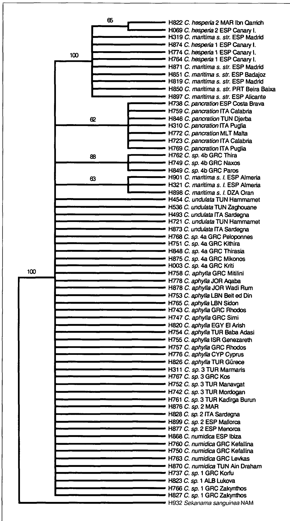
Abb. 46: Strict-Consensus-Tree der Gat- tung Charybdis . Als Outgroup wurde die Schwestergattung Sekanama definiert. Bootstrap- Werte > 50% sind oberhalb der Äste angegeben. Die Analyse der Nukleotidsubstitutionen alleine führt zu einer nicht auf- gelösten Polytomie für die mei- sten Sippen.
