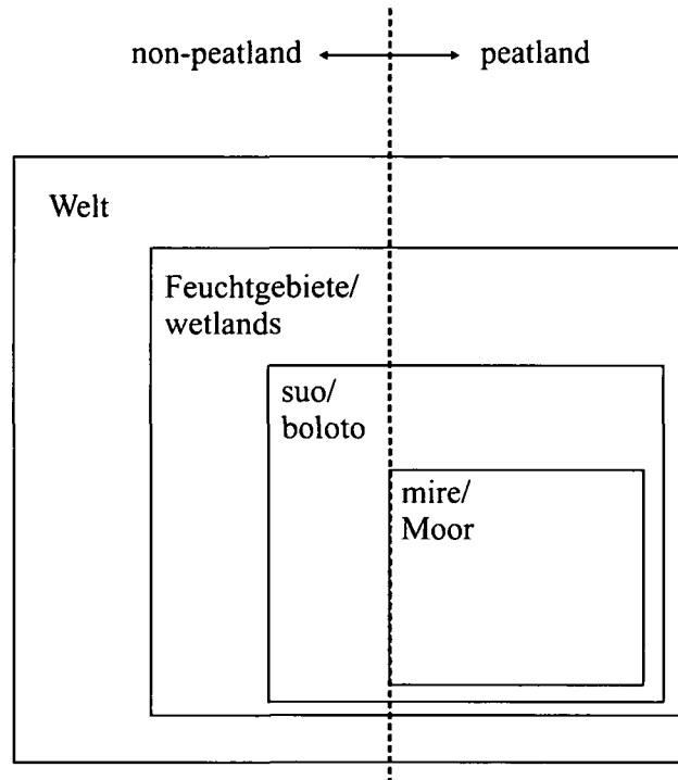
Abb. 1: Die Beziehungen zwischen mire/Moor, suo/bolota, wetland/Feuchtgebiet und peatland. (aus JOOSTEN & CLARKE 2002)
