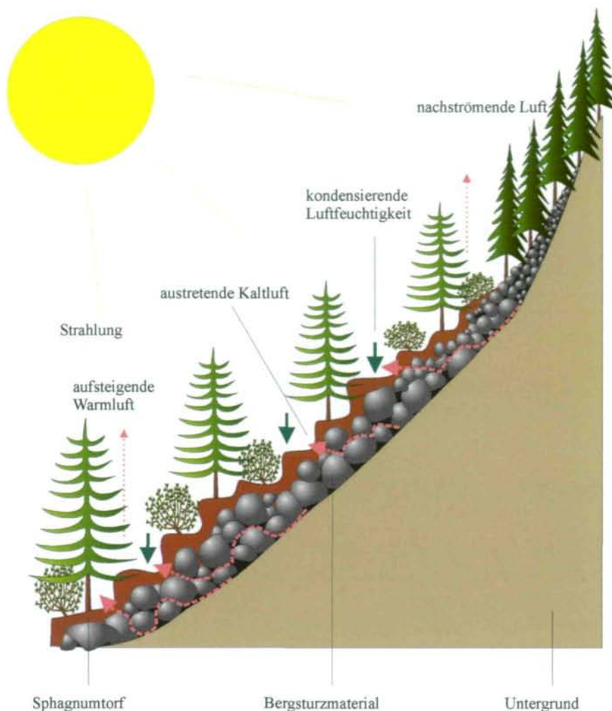
Abb. 51: Schematischer Querschnitt durch ein Kondenswassermoor.
