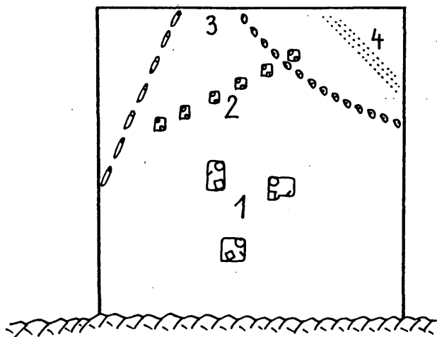
Abb. 1: Schematische Darstellung von Einschlusstypen (Beispiel Fluorit):
