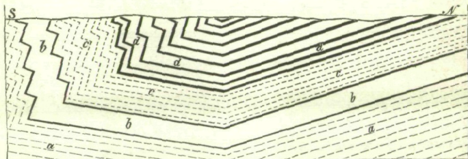
Fig. 3. Ideales Profil der Mulde von Mons. a Devonische Formation. — b Kohlenkalk. — c Flötzleerer Sandstein. — d Productive Kohlengruppe.
