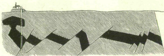
Fig. 2. Vielfach verworfenes Kohlenlager bei Vieille-Pompe in Frankreich.
