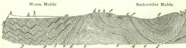
Fig. 4. Profil durch die Worm- und Eschweiler-Mulde. e Devonische Grauwacke. — d Devonischer Kalkstein. — e Unterste subcarbonische Formation. — f Kohlenkalk. — g Productive Kohlenformation. — h Braunkohlen- formation.
