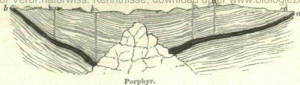
Fig. 1. Querschnitt der Kohlenmulde bei Rive-de-Gier in Frankreich.
