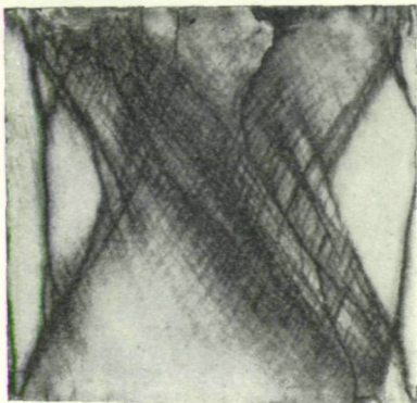
Fig. 5. Carraramarmorwürfel, von oben und unten gedrückt, knapp vor dem Zusammenbruche. Die Risse durch Färbung sichtbar gemacht.
