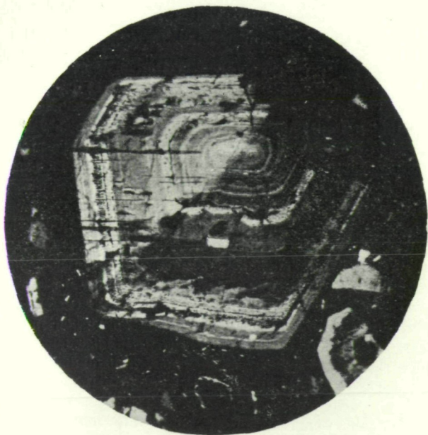
Fig. 6. Kleingefüge von Hornblendeandesit aus Ungarn. Sehr schön zonar gebauter, in Zersetzung befindlicher Feldspat (Plagioklas). Die größtenteils glasige Grundmasse ist auch zersetzt.
