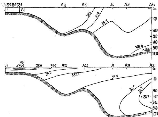
Fig. 2. Vertikale Verteilung des Salzgehalts in der Längsachse der Adria: a) im Februar-März b) im August-September 1912, dargestellt auf Grund der Beobachtungen S. M. S. „Najade“.
