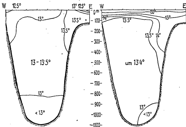
Fig. 4. Verteilung der Temperatur im Querprofil Brindisi—Cap Rodoni (bei Durazzo) a) am 26. Februar 1912, b) am 24. August 1912.
