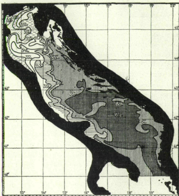
Fig. 1. Salzgehalt an der Oberfläche der Adria im August-September 1911.
