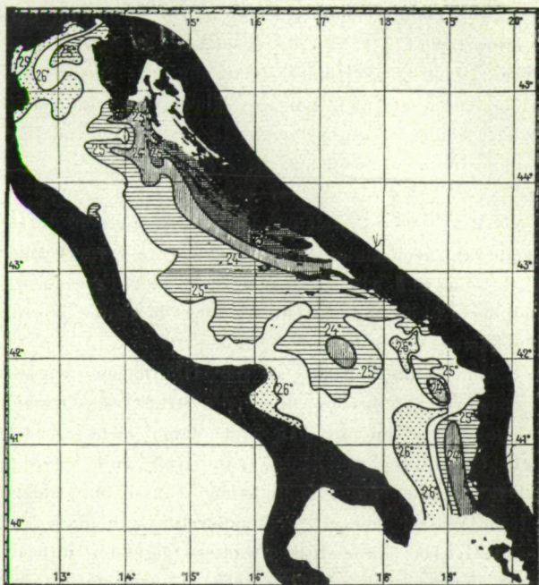
Fig. 3. Temperatur an der Oberfläche der Adria im August-September 1911.
