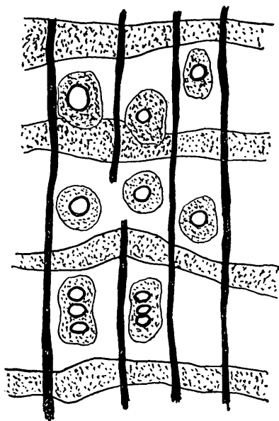
Abb. 4. Holzquerschliff zeigt Gefäße von einem Saum paratrachealen Parenchyms umgeben, „Parenchymaugen“ in der Mitte der Zeichnung. Paratracheales Parenchym kann auch mehrere Gefäße gemeinsam einschließen, wie im Bilde unten sichtbar. Metatracheale Binden durchziehen querverlaufend den Holzkörper und fließen auch häufig mit dem paratrachealen Parenchym zusammen, wie im oberen Teil der Skizze gezeigt wird.
