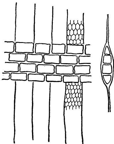
Abb. 1. Homogener Markstrahl, links im Radialschnitt rechts im Tangentialschnitt, als einreihige Spindel erscheinend. Im Radialschnitt verläuft senkrecht auf den Markstrahl ein Tüpfelgefäß.
