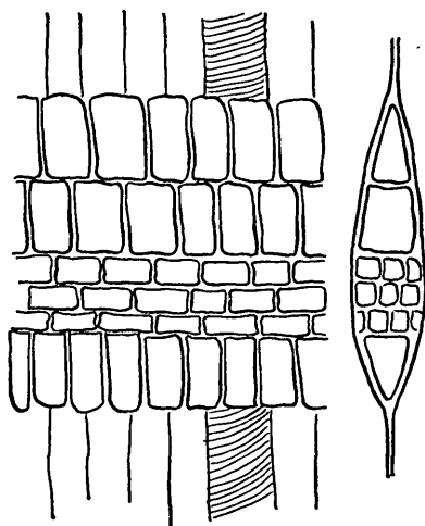
Abb. 2. Heterogener Markstrahl, links im Radialschnitt, rechts im Tangentialschnitt erscheinend. Der Radialschnitt zeigt deutlich oben zwei Reihen von Kantenzellen, unten nur eine solche Reihe, und in der Mitte drei Reihen liegender Zellen.
