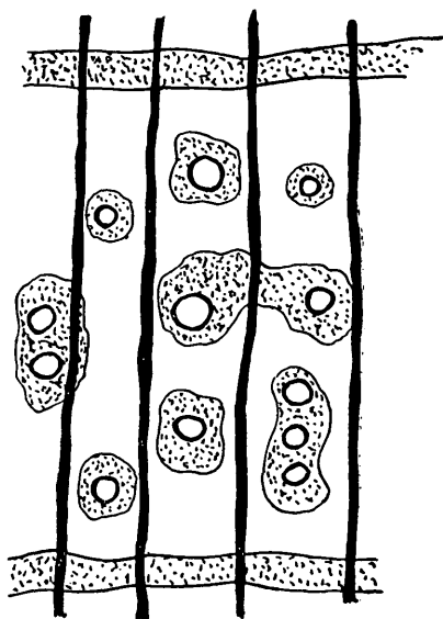
Abb. 5. Holzquerschliff mit paratrachealem Parenchym um die Gefäße und mit „endständigem“ Parenchym oben und unten als querverlaufende Binden zu sehen.
