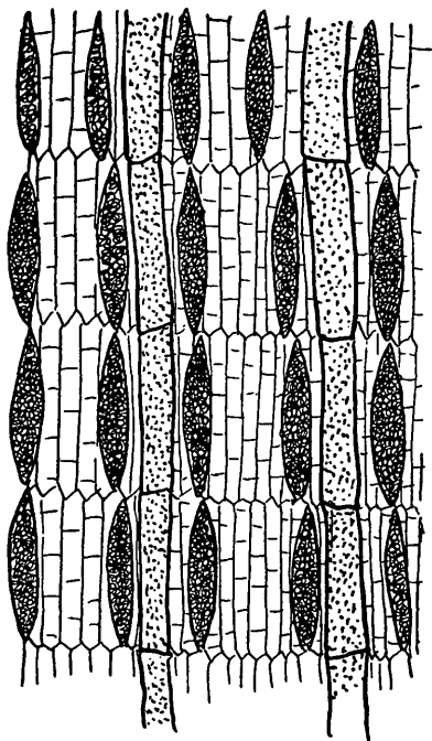
Abb. 3. Stockwerkbau der Markstrahlen, des Holzparenchyms und der Gefäßglieder. Die Markstrahlen erscheinen in der Zeichnung als schmale ovale Spindeln. Zwei Tüpfelgefäße mit stockwerkartig angeordneten Gliedern verlaufen von oben nach unten in der Skizze. Die dünnwandigen Zellelemente sind die Holzparenchymzellen (Tangentialschliff).
