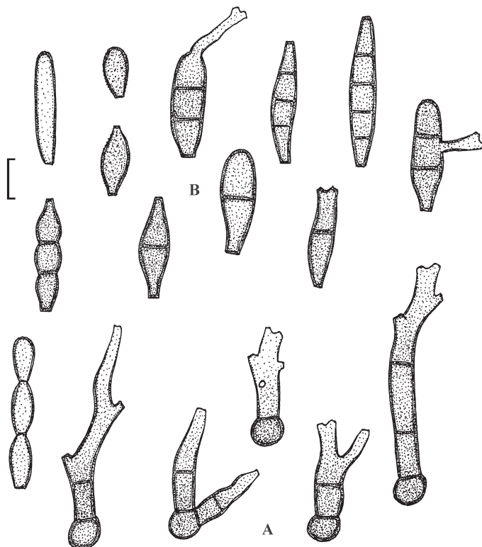
Fig. 3: Fusicladium variabile . A – conidiophores, B – conidia. Bar = 10 \mu m (U. Braun del).
