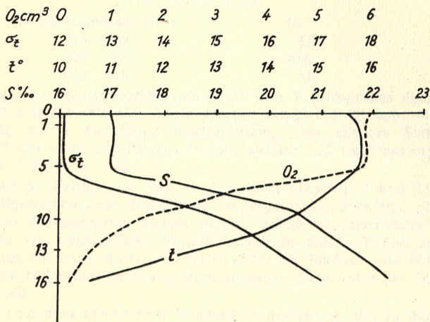
Abb. 1. Stabile Wasserschichtung in der Flensburger Innenförde. „Süd-fall“. Station 132. 29. 9. 1947 ( 54^\circ 21,2'N , 9^\circ 31,0'O ) (nach JARKE 1948)
