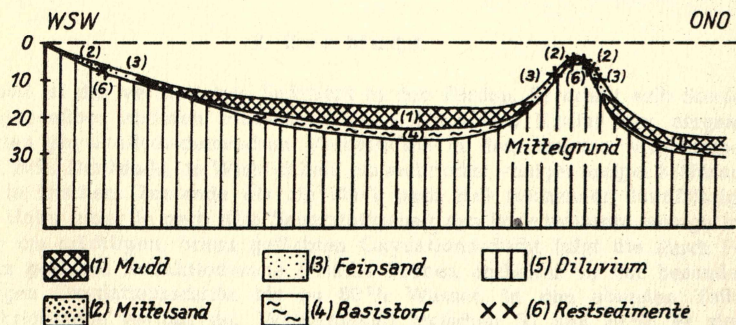
Abb. 2. Schematisches Profil durch die Sedimente der Eckernförder Bucht
