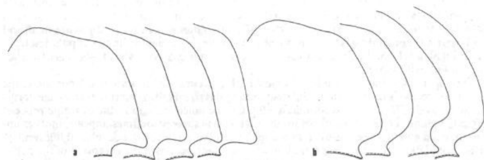
Fig. 23. Ctenophthalmus nifetodes ssp., outline of sternum VIII of males: a. C. n. dzukici ssp. n., paratypes, Jelovica Mt., Bjelasica Mts., Montenegro, b. C. n. martinorum SMIT, Popova Šapka, Šar planina, Macedonia.
