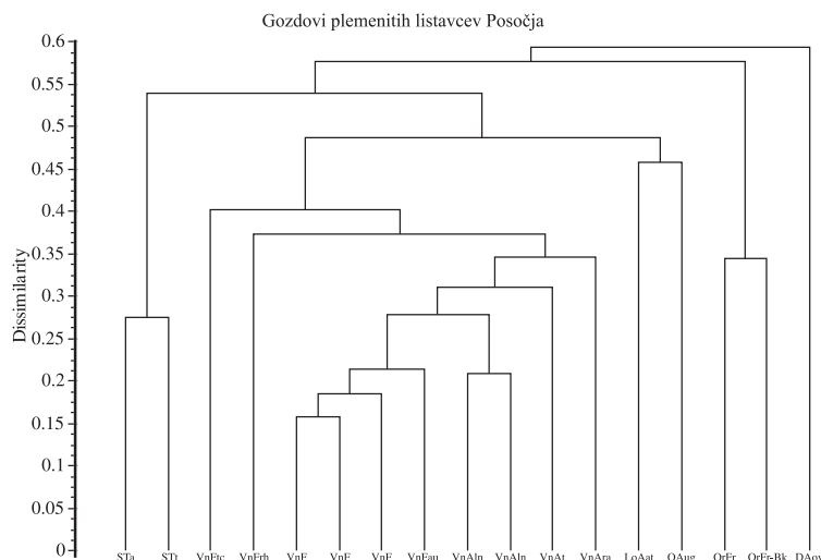
Slika 15: Dendrogram združb plemenitih listavcev v Posočju (UPGMA, similarity ratio).
