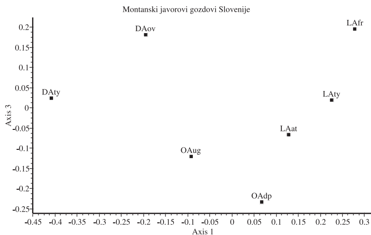
Slika 9: Dvoražsežni ordinacijski diagram nekaterih montanskih združb gorskega javorja v Sloveniji (PCoA, similarity ratio).
