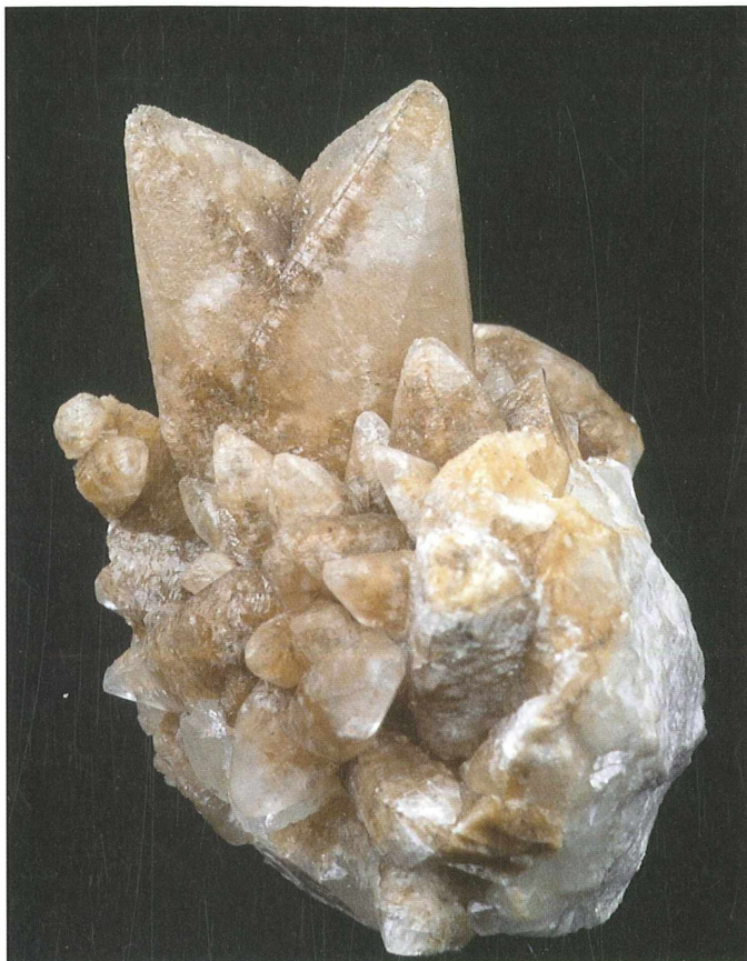
Dvojček skalenoedrskih kristalov kalcita z dvojčično ravnino (021); 40 x 25 mm. Najdba in zbirka Vilija Rakovca. Foto: Ciril Mlinar
