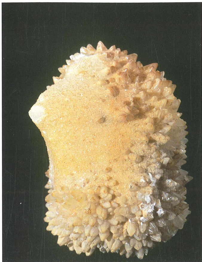
Skupki skalenodrskih kristalov kalcita lahko sestavljajo zanimive oblike; 45 x 55 mm. Najdba in zbirka Zmaga Žorža. Foto: Ciril Mlinar
