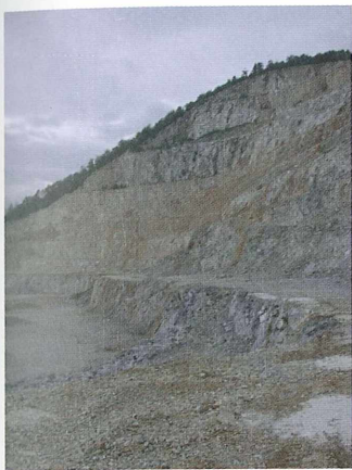
Pogled na del kamnoloma Velika Pirešica leta 2003. Foto: Miha Jeršek
