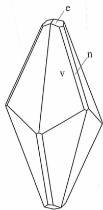
Značilni kristali kalcita iz Velike Pirešice. Skalenodru v\{211\} (A) se pridružujeta romboedra e\{012\} in n\{021\} (B). Risbi: Miha Jeršek
