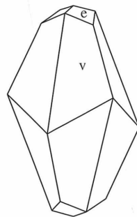
Kristali kalcita z razvitimi skalenoodri v\{211\} in položnimi negativnimi romboedri e\{012\} . Risbi: Miha Jeršek
