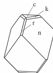
Posebnost kristalov kalcita izpod Stegovnika so kristali z razvitimi kristalnimi ploskvami pinakoida c\{001\} . Na kristalih pa lahko opazimo še kristalne ploskve romboedrov n\{021\} , r\{101\} in k\{011\} . Risbe: Miha Jeršek
