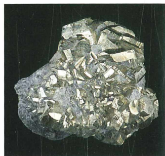
Kristali pirita v glinavcu iz Dolžanove soteske; 30 x 27 mm. Najdba in zbirka Gorana Schmidta. Foto: Ciril Mlinar
