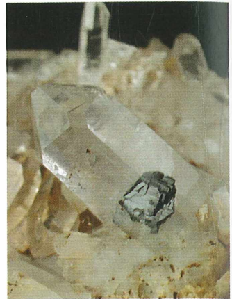
4 mm velik kristal brookita je delno vraščen v kremenu. Dobro vidna je značilna narebrenost na široki ploskvi pinakoida {010}. Najdba in zbirka Vilija Rakovca. Foto Miha Jeršek.
