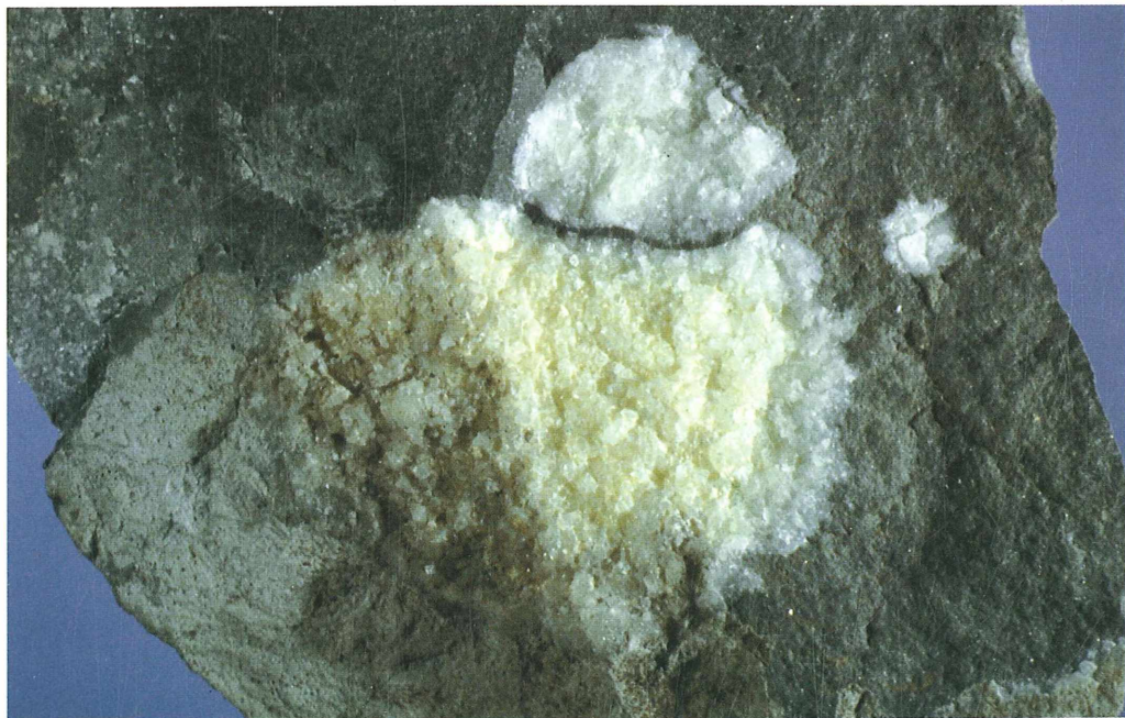
Presek permskega polža iz Račeve pri Žireh, zapolnjenega s kristali kalcita in žvepla; polž 37 x 35 mm. Zbirka Vasje Mikuža. Foto: Marijan Grm
