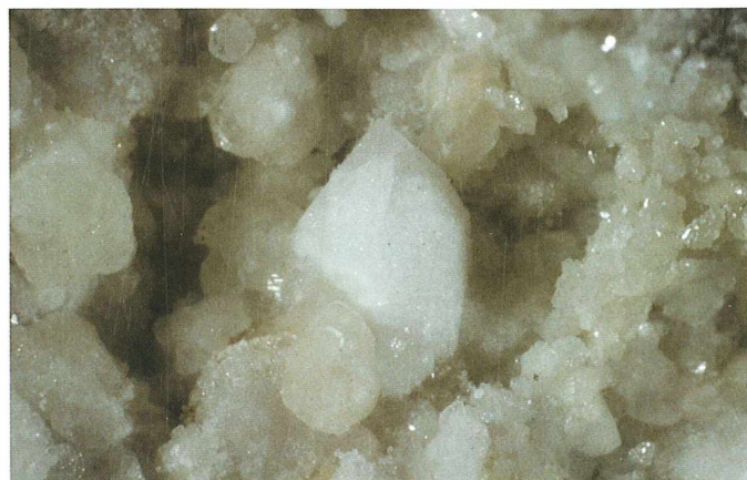
Kristal mlečnega kremen iz Račeve pri Žireh v združbi s kalcitom in žveplom; kremen 5 x 3 mm. Zbirka Vasje Mikuža. Foto: Marijan Grm
