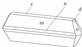
Kristal zoisita z nahajališča Prickler Halt s Svinje/Sauvalpe v Avstriji, kjer je bil odkrit. Pinakoid c\{001\} , prizme d\{012\} , m\{401\} in n\{601\} ter bipi-ramida o\{111\} . Risba: Mirjan Žorž
