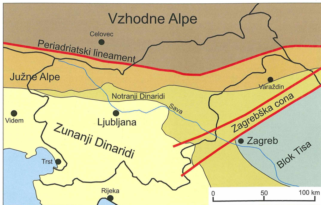
Poenostavljena geotektonska karta Slovenije (po PLACER, 2008, in HERLEC & HLAD, 2005).
