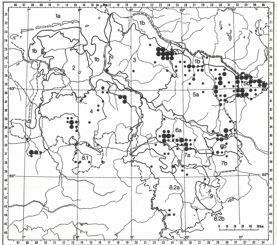
Naturräumliche Regionen
