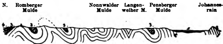
V. Profil der durch Bergbau direkt aufgeschlossenen oberoligocänen und untermiocänen Schichten bei Pensberg. 1) Aeltere Schichten der oberoligocänen Molasse; 2) jüngere Schichten der oberen oligocänen Molasse; 3) untere miocäne Meeresmolasse; 4) jüngere miocäne Molasse.
