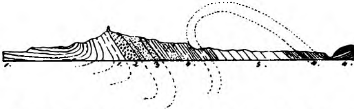
III. Profil durch die oberoligozänen und miocänen Schichten am hohen Peissenberg (1:50000). 1) Obere Süßwassermolasse; 2) Conglomerat derselben; 3) Zwischenregion mit einer Lage der Ostrea crassissima ; 4) Cyrenenmergel mit Pechkohlenflötzen; 5) ältere brackische Molasse.
