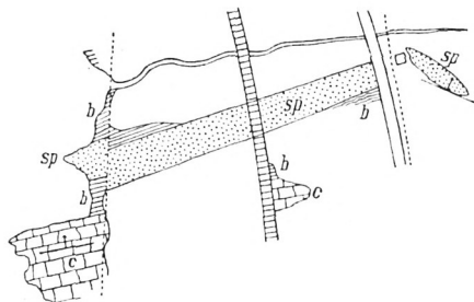
Fig. 12. Links das Seeufer, rechts die Fahrstrasse Moelven-Ring, in der Mitte die Eisenbahnlinie, im Norden der Smedstadellen. sp Sparagmit, c Quarzsandstein, b Birikalk. Die zwei N-S gerichteten punktierten Linien Querverwerfungen.
