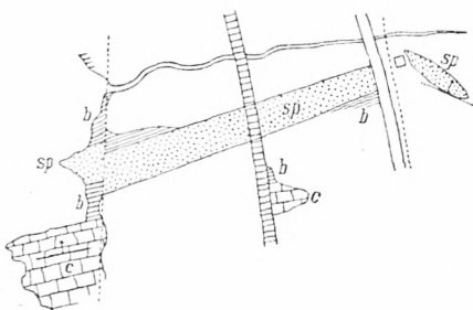
Fig. 4. Links das Seeufer, rechts die Fahrstrasse Moelven-Ring, in der Mitte die Eisenbahnlinie, im Norden der Smedstadelven. sp Sparagmit, c Quarzsandstein, b Birikalk. Die zwei N-S gerichteten punktierten Linien Querverwerfungen.
