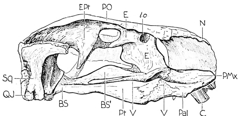
Fig. 15. ? Cryptocynodon spec. Exemplar und Fundort wie Fig. 10. — Schädel von rechts her aufgebrochen, um die Elemente der Sagittalebene zu zeigen. — Nat. Gr.
