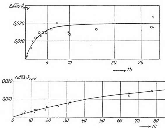
Abb. 16. Die reversible \overline{\cos \vartheta} -Änderung beim Wechsel 11^\circ - 99^\circ - 11^\circ C in Abhängigkeit von der Feldstärke
