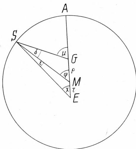
Fig. 2. Exzenter mit Ausgleichspunkt G
