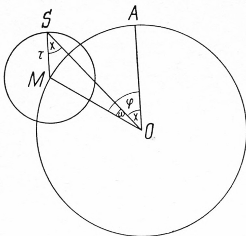
Fig. 1. Epizykel
