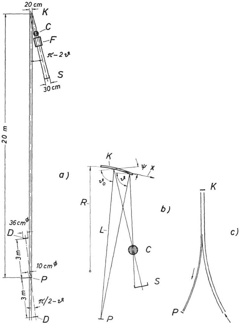
Abb. 1a. Laufzeitfokussierung für Neutronen von 600 m/sec durch einen parallel schwingenden, ebenen Kristall. K = Kristall ((111)-Ebene von Si ). Schwingungsfrequenz 100/sec, Amplitude 4,6 cm. P = Probe, 0,1 cm dick; D = Detektoren; C = Hilfschopper, Öffnungszeit 480 \mu sec; S = Strahlrohrende am Reaktor; \theta = Braggwinkel.
