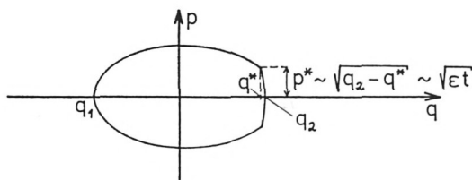
Fig. 2: Verhältnisse für den Fall, daß sich Diskontinuität und Umkehrpunkt mit einer Geschwindigkeit der Ordnung \varepsilon voneinander entfernen.
