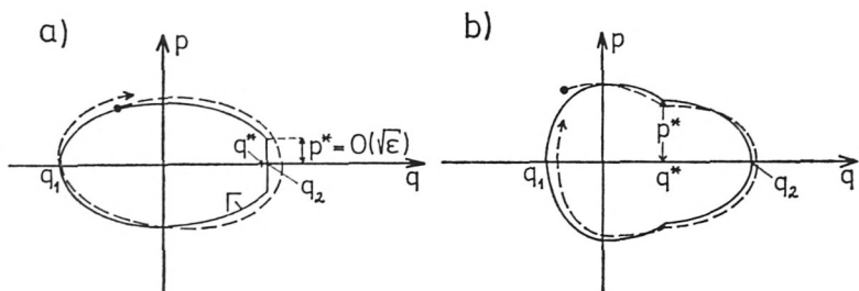
Fig. 1: Charakteristische eingefrorene (ausgezogen gezeichnet) und wirkliche Teilchenbahnen in der Phasenebene bei sprungartiger Änderung der Kräfte um die Ordnung 1.
