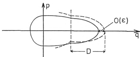
Fig. 3: Eingefrorene und wirkliche Teilchenbahnen in der Phasenebene bei Änderung der Kräfte um die Ordnung 1 über Strecken der Größenordnung D
