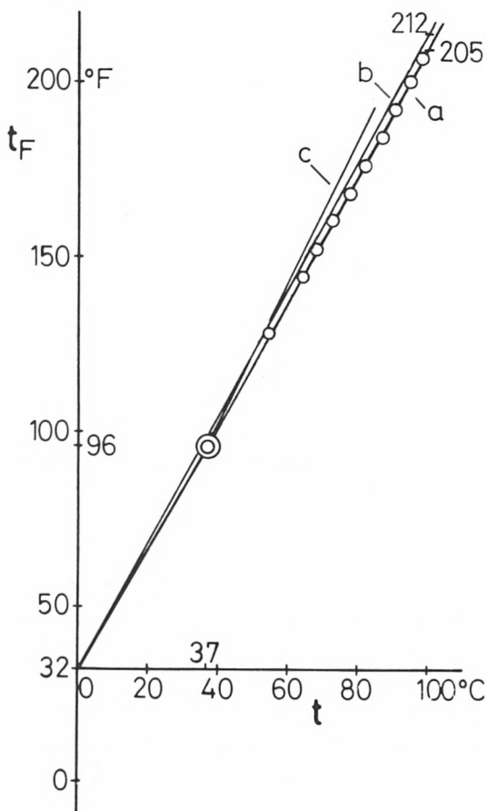
Bild 11: t_{\text{F}}, t -Diagramm mit den Dampfdruckmessungen Fahrenheits (Kreise). Gerade a für t'_{\text{F}} = 205^{\circ}\text{F} , Gerade b für t'_{\text{F}} = 212^{\circ}\text{F} , Kurve c extrapolierte Weingeistskala.
