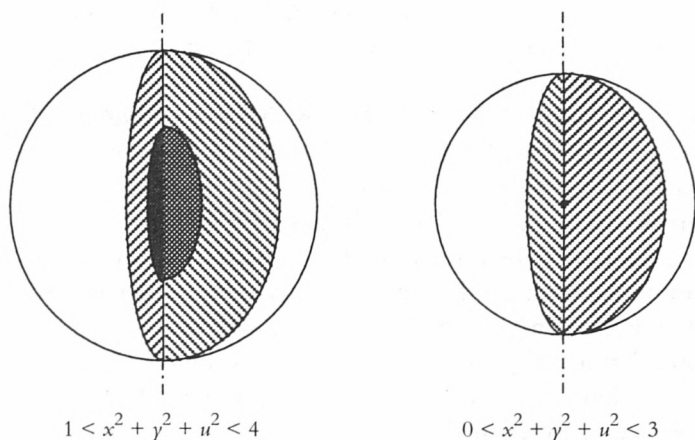
Abb. 1 Schnitte \nu = 0 (links) und \nu = 1 (rechts) der Hypersphärenschele 1 < |x + iy|^2 + |u + iv|^2 < 4
