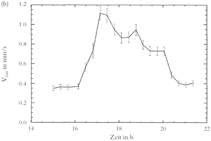
Abbildung 7: (a) Protokoll eines Beleuchtungsexperiments einer Maispflanze im NMR-Magneten. Die Beleuchtungsstärke wurde um 16.30 Uhr auf 950 \mu\text{E} eingestellt und danach im 1-Stunden-Intervallen stufenförmig abgeschaltet. (b) Die Flussgeschwindigkeit von Wasser in den Xylemgefäßen der Maiswurzel wurde mit bildgebenden NMR-Methoden bestimmt. Vom Basiswert 0,35 \text{ mm/s} im unbeleuchteten Zustand steigt die Geschwindigkeit auf 1,1 \text{ mm/s} und nimmt anschließend parallel zum Beleuchtungsprotokoll wieder ab.
