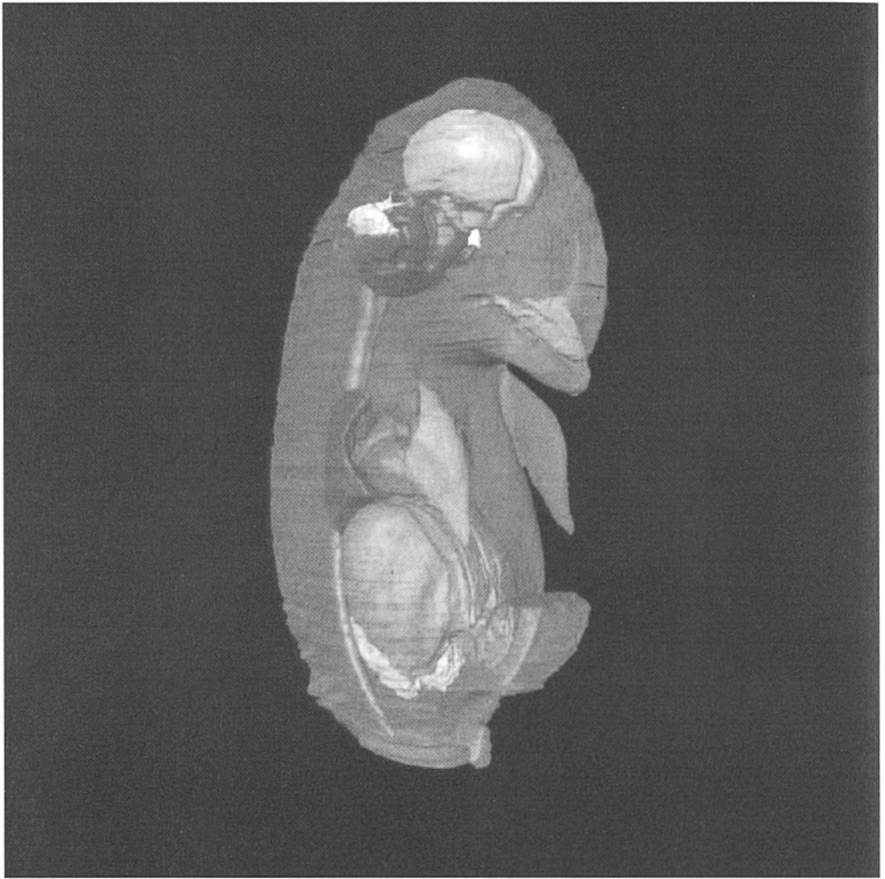
Abbildung 2: Dreidimensionales NMR-Bild eines Delphinembryos. Besonders gut zu sehen sind die inneren Organe (von oben nach unten): Gehirn, Rückenmark, Herz, Leber. Die Messdaten wurden an einem 11.7T NMR-Gerät aufgenommen. Die Ortsauflösung beträgt 100 \mu\text{m} .
