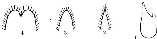
Fig. 1—3. Ungefähre Umrissfiguren der Hüllspelzenendigungen.
