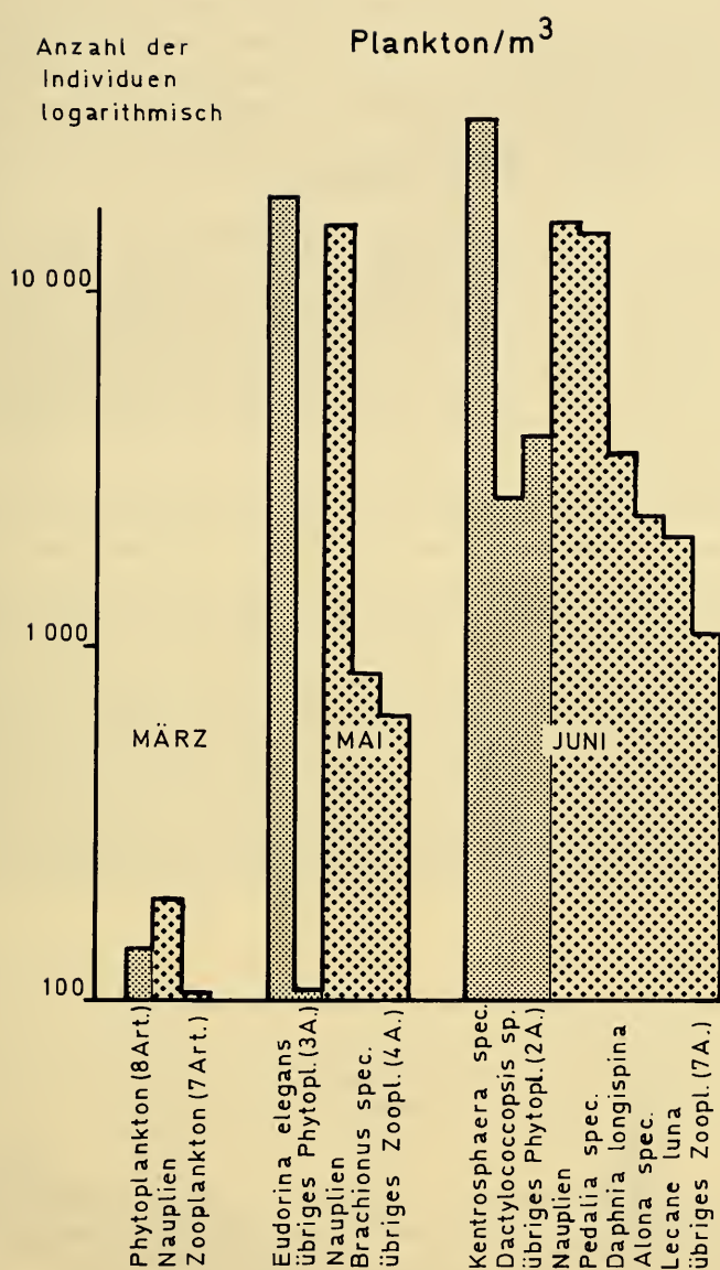
Abb. 8: Netzplankton-Verteilung
