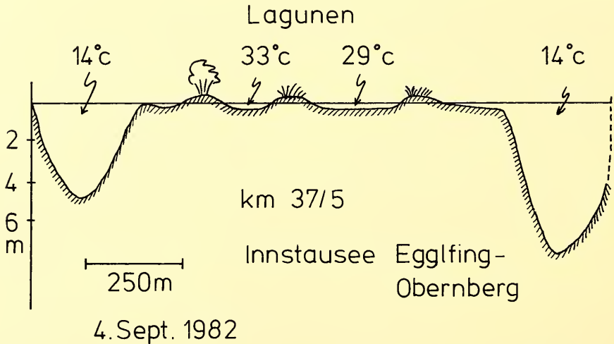
Abb. 1: Querschnitt durch die Insel im Stauraum Eggfing-Obernberg am unteren Inn bei Flußkilometer 37/5 mit der Verteilung der Wassertemperaturen am 4. September 1982 (14 Uhr). Die als „Lagunen“ bezeichneten, flachen Restwasserflächen auf der zentralen Insel beherbergten das Massenvorkommen von Heterocypris incongruens und waren das Zentrum des Botulismus-Ausbruchs. – Cross-section through the Eggfing-Obernberg impoundment on the lower Inn river at the place of the outbreak of botulism. Water temperatures were taken on September 4, 1982 at 2.00 p.m. The shallow ‘lagoons’ of freshwater contained the population of the ostracod Heterocypris incongruens .
