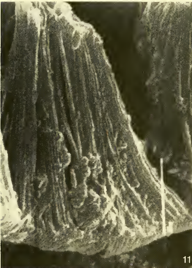
Abb. 9–11: Anolis equestris (s. Abb. 7). 9: Dünnes Endglied der Zehe von unten gesehen, seitlich drei Borstensinnesorgane. Die Rauigkeit der Oberfläche wird durch einen Borstenbesatz bedingt. 10: Haftlamellen des verbreiterten Zehenteils (vgl. Abb. 13). Es ist unklar, ob es sich bei der Aufwölbung und dem Einreißen der Lamellenkanten und der in Abb. 12 besonders deutlichen Verschmelzung der Borsten um ein konservierungsbedingtes Artefakt handelt oder möglicherweise ein Vorbereitungsstadium der Häutung vorliegt, wobei jedoch die Untersuchungen zweier Individuen gleiche Ergebnisse lieferten. In anderen ebenso konservierten Präparaten (z. B. Abb. 19, 22) sind diese Strukturen jedoch bis ins kleinste Detail erhalten, so daß daraus möglicherweise auch taxonomische Schlußfolgerungen zu ziehen wären. 11: Distaler Bereich der Borsten von Abb. 10. Haftborsten von 30\mu Länge (die Messung stimmt mit der lichtmikroskopischen Bestimmung von RUIBAL & ERNST, 1965, genau überein). – Abb. 12: Anolis concolor , ZSM 383/81. Deutlich sind einige freistehende Setae mit ihren Spatulae zu erkennen.
