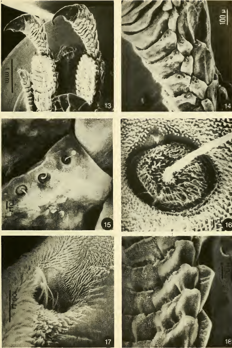
Abb. 13–18: Anolis cybotes . 13: Übersichtsaufnahme, auf welcher der Gegensatz zwischen dem verbreiterten, mit Haftborsten versehenen Zehenteil und dem hochgewölbten Endstück gut zu erkennen ist. Der Zustand ist konvergent zu den morphologischen Verhältnissen der Geckonidengattung Hemidactylus (Halbfinger) (s. SCHLEICH & KÄSTLE 1984). 14: Ausschnitt aus dem distalen, krallentragenden Teil der Zehe von Abb. 13. Sämtliche Schuppen tragen randständige Borstensinnesorgane. 15: Ausschnitt aus Abbildung 14. Die unterschiedlich hellen Bereiche sind Felder mit verschiedenen großen Borsten. Auf der links oben angrenzenden, relativ dunklen Schuppe sind möglicherweise Zellen zu sehen. Die verschiedenen hellen Borstenfelder decken sich vermutlich nicht mit Zellengrenzen. 16: Ausschnitt aus Abbildung 15, borstentragendes Sinnesorgan. Die Borsten der angrenzenden Haut sind an der Basis 0,3 \mu dick und etwa 1 \mu lang. 17: Ausschnitt aus einer lateralen Schuppe aus Abb. 14. Das Sinnesorgan trägt mehrere Borsten, und die angrenzende Schuppenoberfläche ist glatt. 18: Ausschnitt aus dem verbreiterten Zehenteil von Abb. 13. Der Borstenbesatz zieht sich auch über den Seitenrand der Lamelle hin. Hier, wie auch an der Basis der Lamellen, sind die Borsten kurz und bilden einen samtigen Überzug. Auf den drei Randschuppen stehen zahlreiche Borstensinnesorgane.
