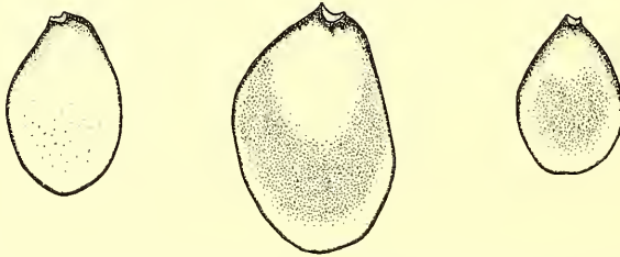
Abb. 1: 1., 4. und 7. Kieme der Larve von Baetis lutheri Müller-Liebenau.
