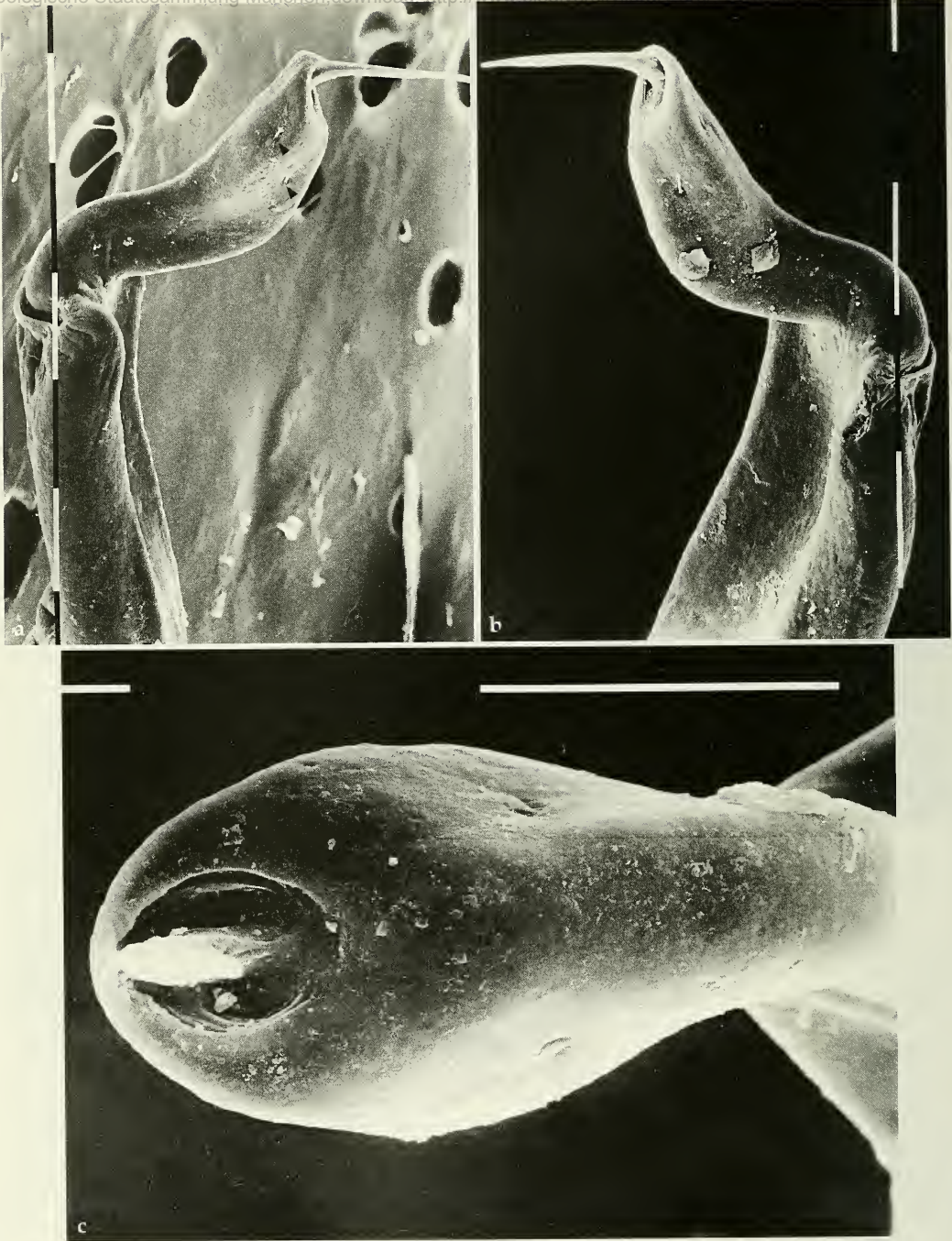
7. Graecophalangium drenskii , spec. nov., Holotypus ♂. Glans penis, REM-Aufnahmen: a. lateral, × 203 (Pfeile: Börstchen); b. lateral, × 252; c. dorsal, × 500. Skalen: 100 µm
