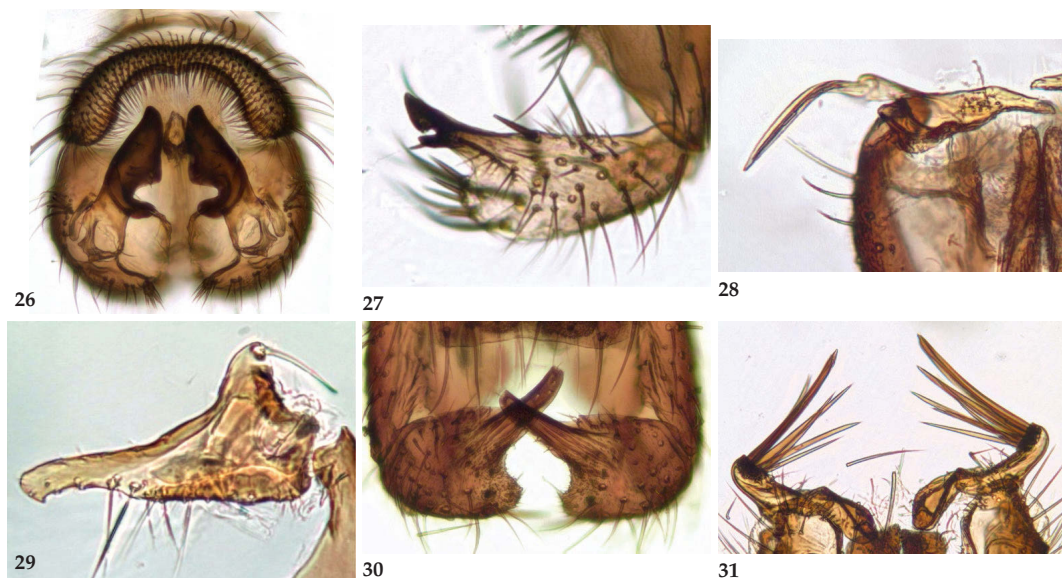
Fig. 26–31. Gonostyli. 26. Tetragoneura caliga . 27. T. caligula . 28. T. lustra . 29. T. dixie . 30. T. canada . 31. T. polyspina .
