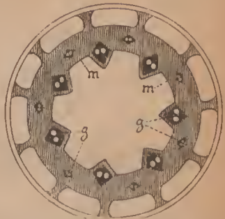
Fig. 2. Querschnitt durch den Halm von Molinla coerulea : m mechan. Gewebe, g Gefässbündel. Schematisch. (Nach Kerner.)
