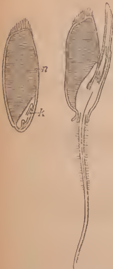
Fig. 8. Längsschnitt durch ein Weizenkorn vor und nach der Keimung: n Nährgewebe, k Keim. 4fache Vergr. (Nach Körner.)
