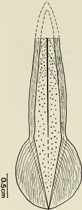
Abb. 2. Libanoteuthis libanotica (FRAAS 1878), Obercenoman von Hakel, Rekonstruktion des Gladius. Das fehlende Stück des vorderen Endes wurde ergänzt (gestrichelte Linie).
