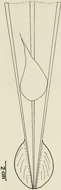
Abb. 1. Dorateuthis sabilalmae (NAEF 1922), Obersanton von Sahil Alma, Rekonstruktion des Gladius und angegebener Position des Tintenbeutels. Die Proportionen der Konusfahnen sind nicht ganz sicher. Die Form des vorderen Randes ist ebenfalls unsicher.
