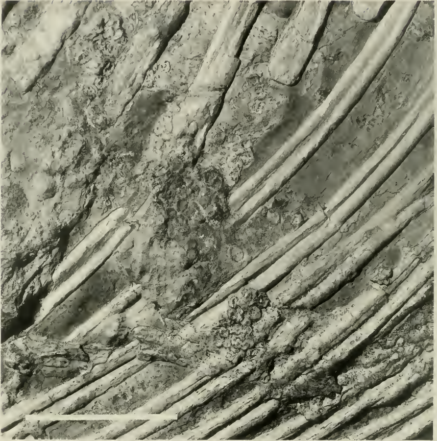
Abb. 15. Ausschnitt aus dem Rumpfbereich des in Abb. 1 gezeigten Skeletts mit zahlreichen kleinen Wirbeln. Am linken Bildrand ist das vordere Ende der Häkchenverballung zu erkennen. M = 10 cm.
