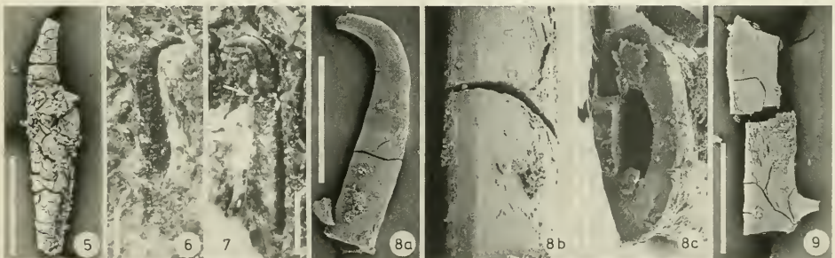
Abb. 5–9. Cephalopodenfanghaken der Formen 1 und 2 aus dem Mageninhalt des in Abb. 1 gezeigten Skeletts. Die in Abb. 5, 8 und 9 gezeigten Haken sind aus dem Gestein herausgeätzt, die übrigen liegen noch im Gestein.
