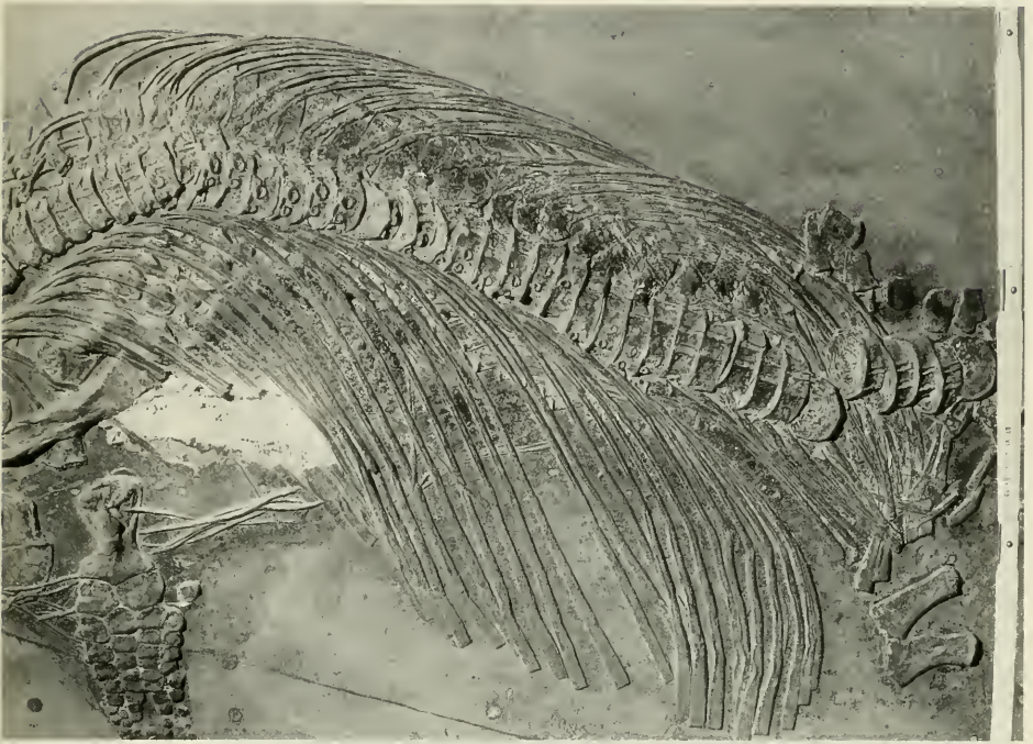
Abb. 16. Stenopterygius sp.; Teil eines Skeletts aus dem Schwarzjura \epsilon II, von Holzmaden, Inv.-Nr. 54 816; vor 1984 Sammlung ZELLER, Eislungen (v. HUENE 1922: 56). Das Skelett, das lange in einer Garage stand, zeigt einen sehr stark ausblühenden Mageninhalt, der die überlagernden Rippen zum Teil abgesprengt hat. Schräg darüber liegt schwarzer, nicht ausblühender Mageninhalt. Zwischen diesem und der Wirbelsäule liegen einige Wirbel eines Embryos, weiter caudad sind einige kleine Flossenelemente zu erkennen.
