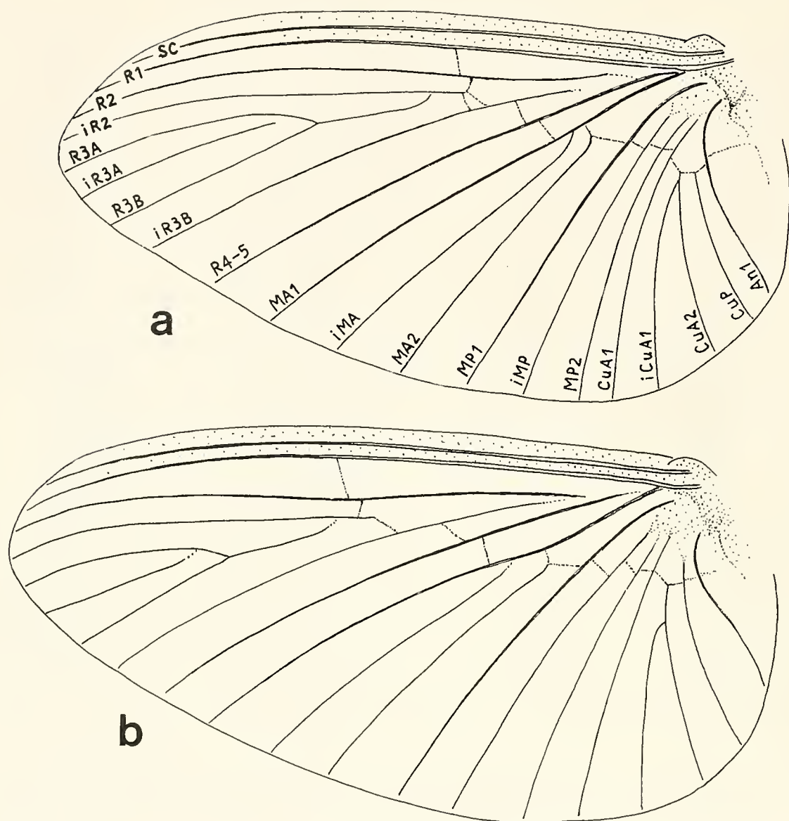
Abb. 5. Flügel. — a. Afrocercus forcipatus , — b. Tasmanocaenis tillyardi . — Flügellänge a: 2,5 mm; Flügellänge b: 3,5 mm.
