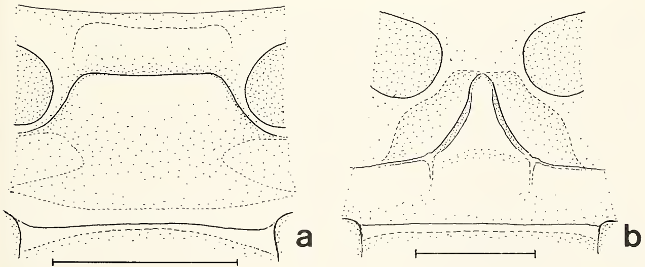
Abb. 4. Mediane Partie des Prothorax zwischen den Coxae. — a. Afrocercus forcipatus , — b. Tasmanocaenis tillyardi . — Maßstäbe: 0,2 mm.
