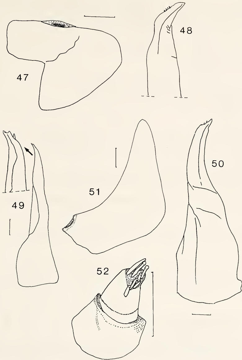
Figs. 47–48. Paraschizidium aegaeum n. sp.; male (holotype) (scale: 0.02 mm). – 47. Pleopod-exopodite I; – 48. Apex of pleopod-endopodite I. Fig. 49. Paraschizidium album n. sp., male (holotype) (scale: 0.02 mm); pleopod-endopodite I (apex enlarged). Figs. 50–51. Paraschizidium falkoneriae n. sp.; male (holotype) (scale: 0.02 mm). – 50. Pleopod-endopodite I; – 51. Pleopod-exopodite II. Fig. 52. Paraschizidium levithae n. sp., female (scale: 0.02 mm); antennula.
