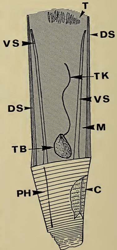
Abb. 1a. Sueviteuthis zellensis n. gen. n. sp., Holotypus. GPIT 1564/1. — x 1.
