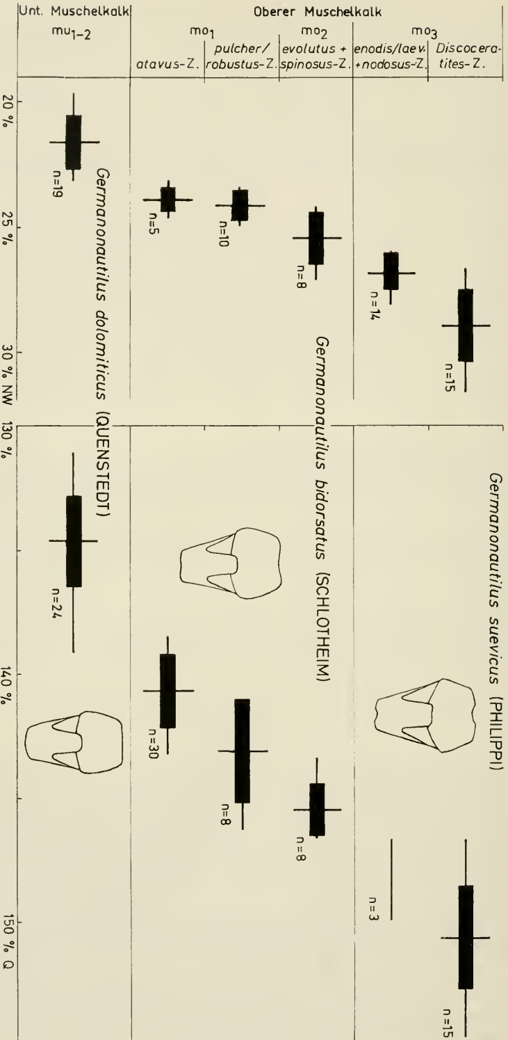
Abb. 5. Phylogenetische Reihe von Germanonautilus im Unteren und Oberen Muschelkalk. Links: Nabelweilen, rechts: Querschnitte. Die Nabelweite nimmt im Laufe der Entwicklung immer mehr zu, und der Querschnitt wird breiter. — Senkrechter Strich: Mittelwert; dicker Balken: Standardabweichung; waagerechter Strich: Variationsbreite.
