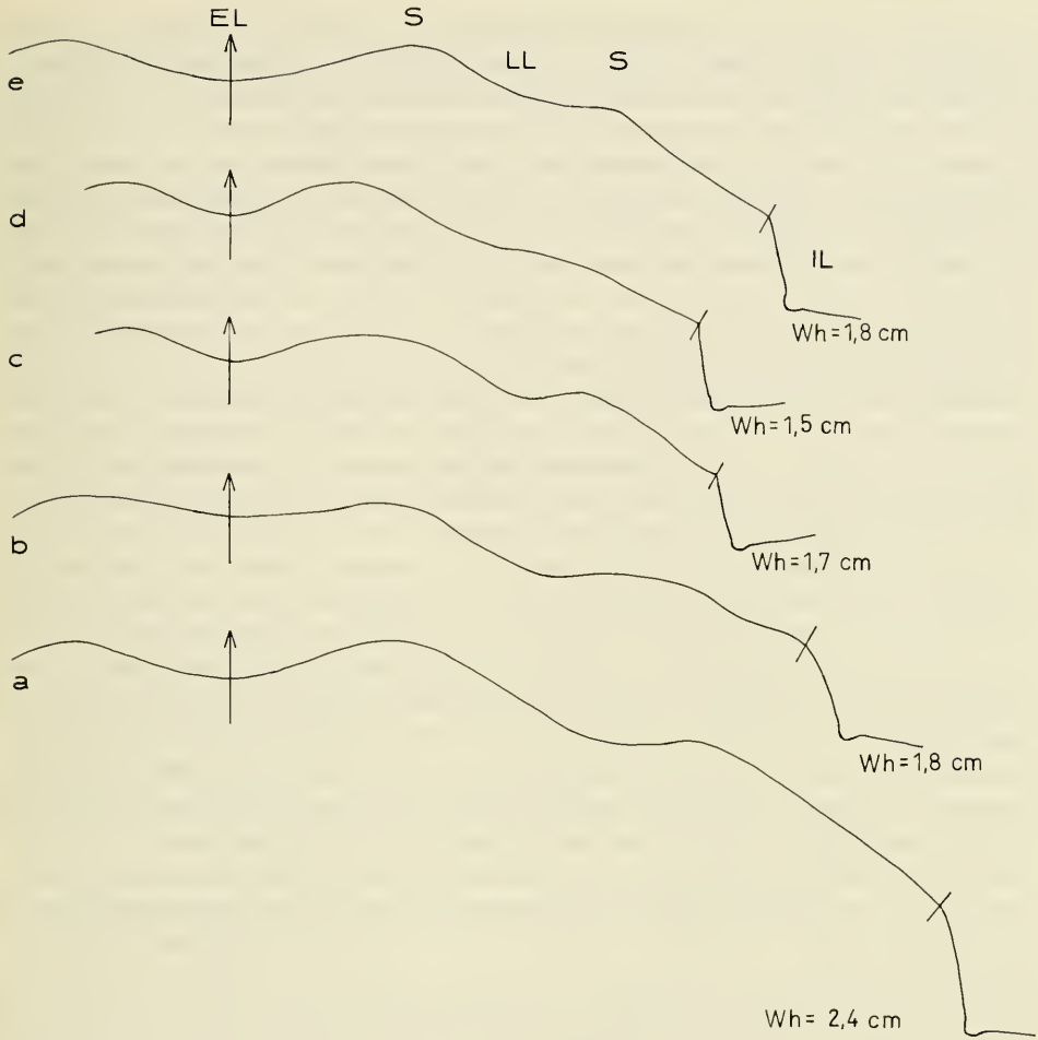
Abb. 2. Lobelinien von Germanonautilus .
