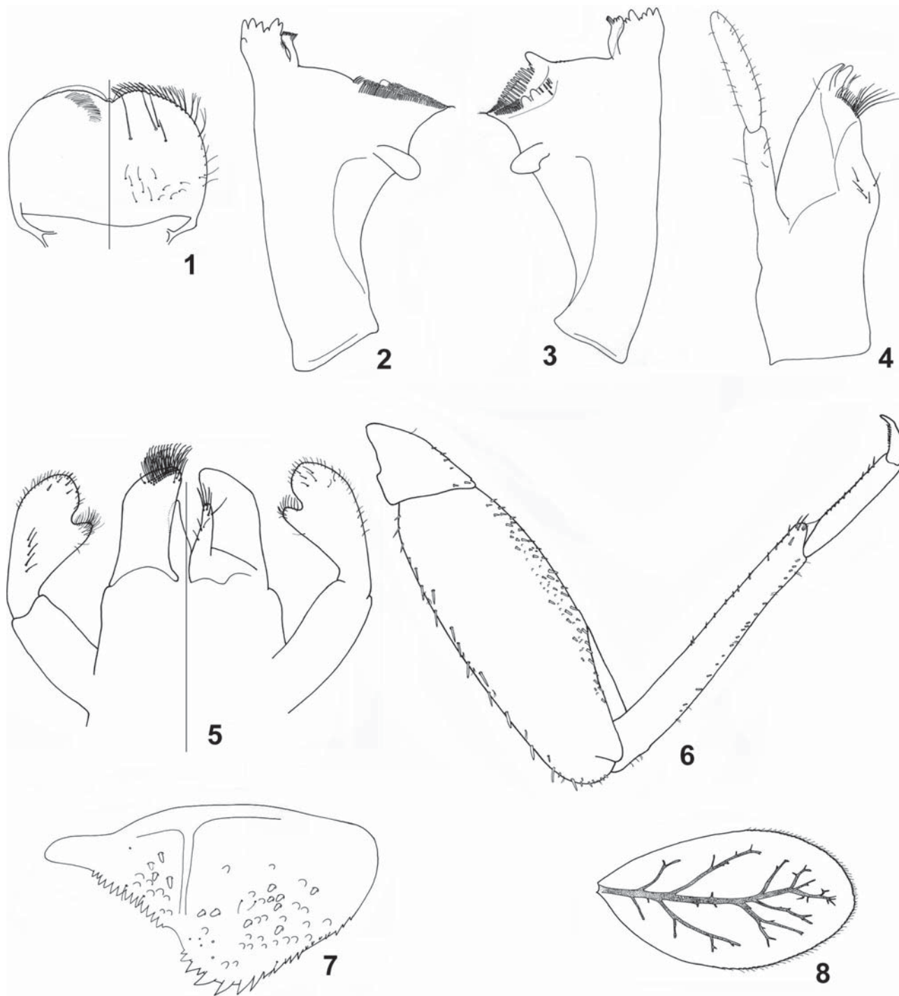
Figs. 1–8. Labiobaetis paradisus n. sp., larva. – 1. Labrum (left half: posterior view; right half: anterior view). 2. Right mandible (posterior view). 3. Left mandible (posterior view). 4. Right maxilla (posterior view). 5. Prementum of labium (left half: posterior view; right half: anterior view). 6. Right foreleg (anterior view). 7. Paraproct. 8. Gill IV.
