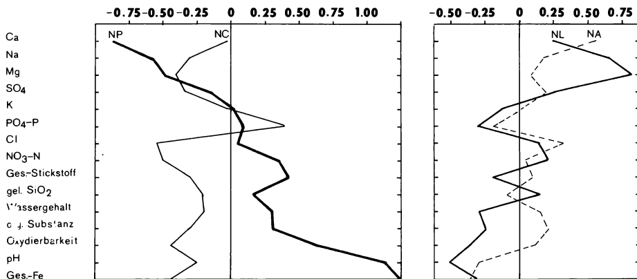
Abb. 4: Vergleich der Bodensubstrate in den untersuchten Gesellschaftstypen mit der Methode der Merkmalslinien. Der pH-Wert wird als spezifische Azidität ausgedrückt.
