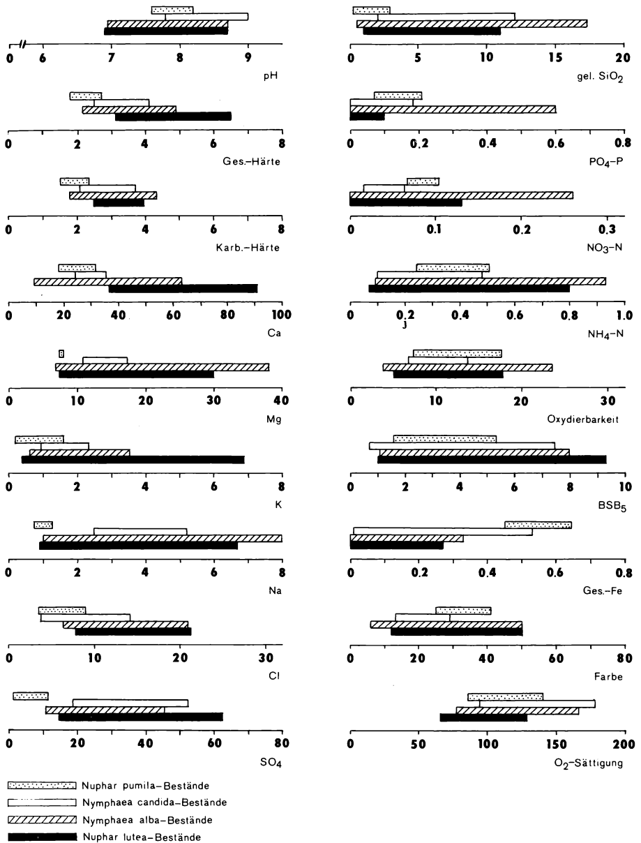
Abb. 3: Bereiche der Wassereigenschaften in den untersuchten Gesellschaftstypen. Die meisten Werte in mg/l außer: pH, Gesamthärte und Karbonathärte (mval/l), Oxydierbarkeit und BSB 5 (mg O 2 /l), O 2 -Sättigung (%).
