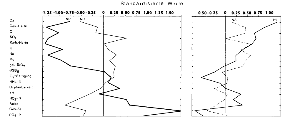
Abb. 2: Vergleich der Wassereigenschaften in den untersuchten Gesellschaftstypen mit der Methode der Merkmallinien. Der pH-Wert wird als spezifische Azidität ausgedrückt.
