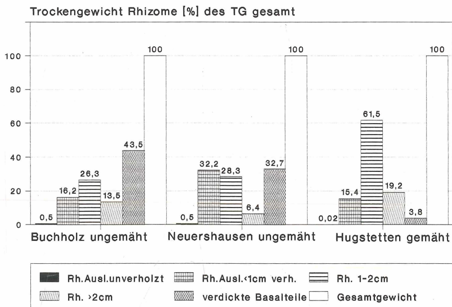
Abb. 5: Verteilung von Rhizomgrößenklassen unter drei Versuchsflächen (s. Text). (a): Trockengewicht der Rhizome in kg/m; (b): in % des Gesamtrockengewichts.
