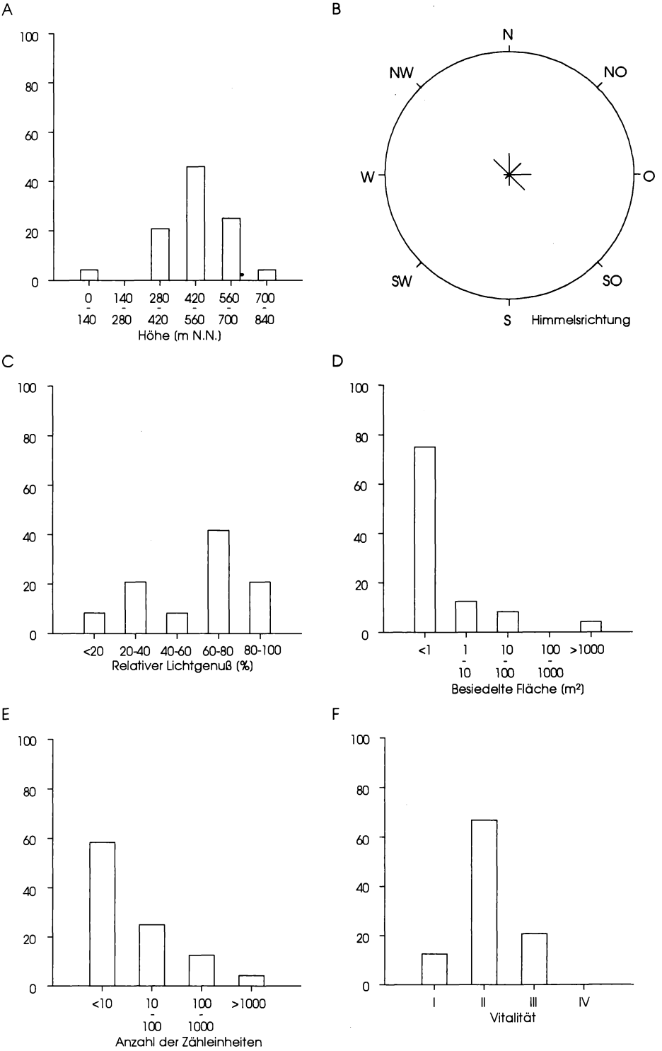
Abb. 7: Standort- und populationsökologische Charakteristika (relative Häufigkeit in %) der nordrhein-westfälischen Vorkommen von Lycopodium tristachyum ; A Höhenlage, B Exposition (Kreisradius entspricht 100%), C relativer Lichtgenuß, D besiedelte Fläche, E Größe und F Vitalität der Populationen.
