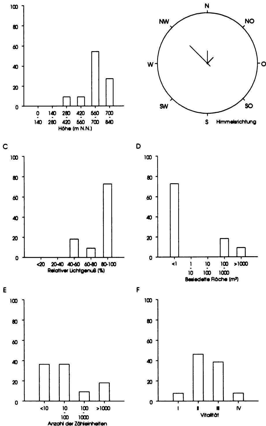
Abb. 8: Standort- und populationsökologische Charakteristika (relative Häufigkeit in %) der nordrhein-westfälischen Vorkommen von Lycopodium alpinum ; A Höhenlage, B Exposition (Kreisradius entspricht 100%), C relativer Lichtgenuß, D besiedelte Fläche, E Größe und F Vitalität der Populationen.
